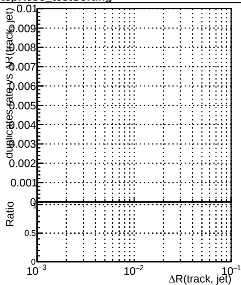
testSorting
