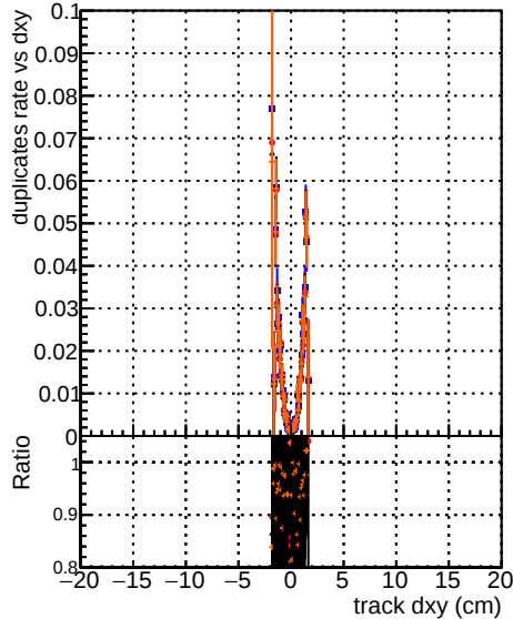
testSorting
