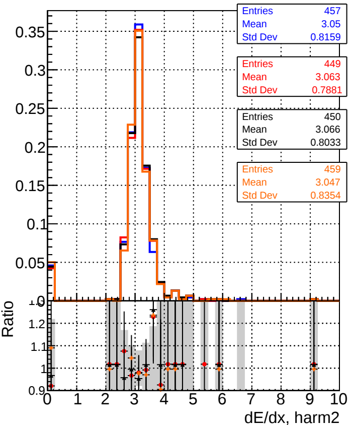
dE/dx estimator 3
