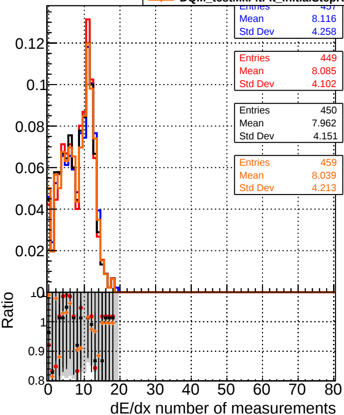
dE/dx estimator 3
