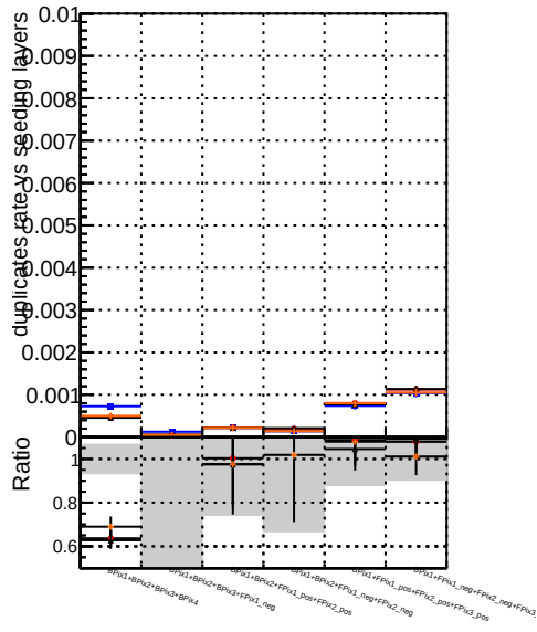
Chi2Zero
