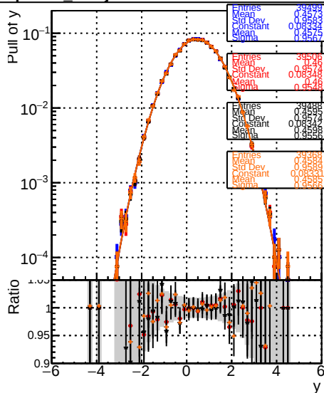
RecoPVAssoc2GenPVMatched_PullY
