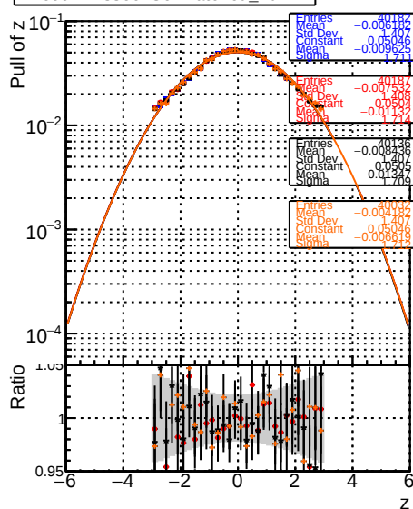
RecoAllAssoc2GenMatched_PullZ
