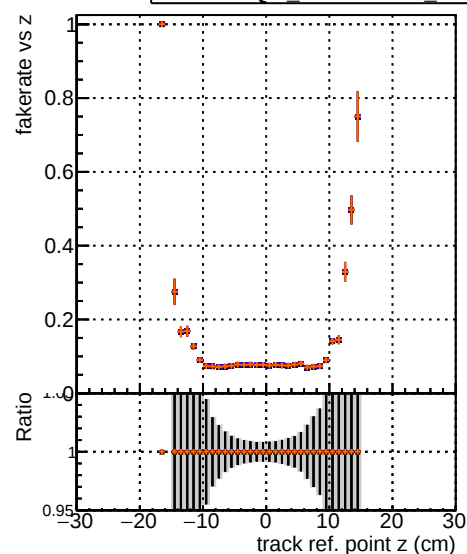
DOM original4 DOM fit4 DOM fit4 initialStepReso DOM fit4 initialStepReso wRejection10
