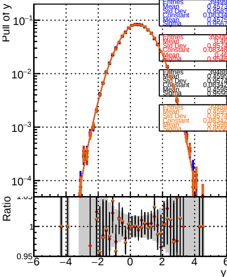
RecoPVAssoc2GenPVMatched_PullY
