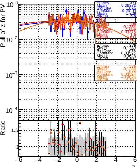
RecoPVAssoc2GenPVMatched_PullZ
