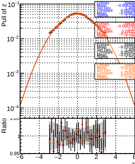
RecoAllAssoc2GenMatched_PullZ
