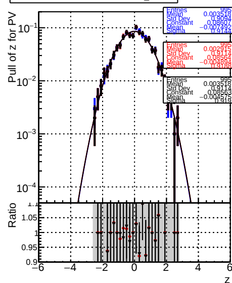
RecoPVAssoc2GenPVMatched_PullZ
