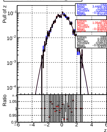
RecoAllAssoc2GenMatched_PullZ
