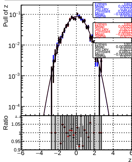
RecoAllAssoc2GenMatched_PullZ
