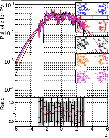
RecoPVAssoc2GenPVMatched_PullZ
