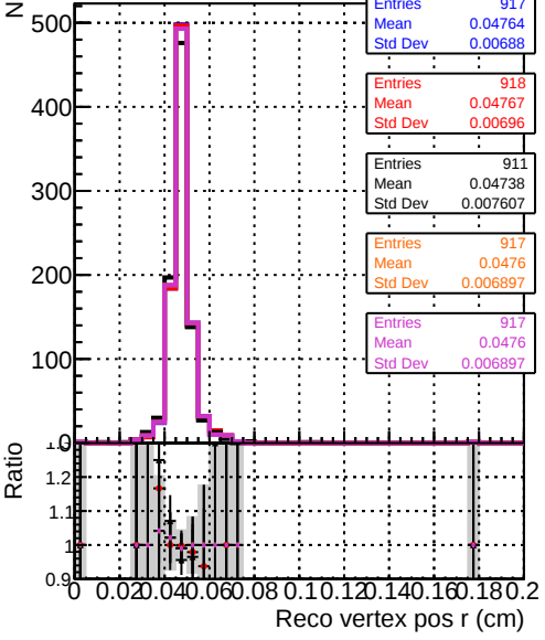
Recons DOM original step2 pt1to20 eta0p0to0p4 DOM angle step2 pt1to20 eta0p0to0p4 DOM fast step2 pt1to20 eta0p0to0p4 DOM mkFit step2 pt1to20 eta0p0to0p4 DOM CPEpixel3 step2 pt1to20 eta0p0to0p4
