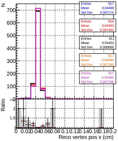
Recons DOM original step2 pt1to20 eta0p0to0p4 DOM angle step2 pt1to20 eta0p0to0p4 DOM fast step2 pt1to20 eta0p0to0p4 DOM mkFit step2 pt1to20 eta0p0to0p4 DOM CPEpixel3 step2 pt1to20 eta0p0to0p4
