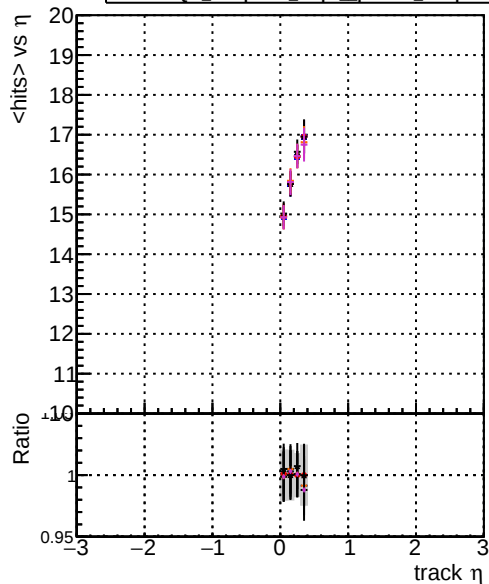
DOM original step2_pt1to20_eta0p0to0p4 DOM angle_step2_pt1to20_eta0p0to0p4 DOM fast_step2_pt1to20_eta0p0to0p4 DOM mkFit_step2_pt1to20_eta0p0to0p4 DOM CPEpixel2_step2_pt1to20_eta0p0to0p4
