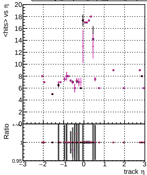
DOM original step2_pt1to20_eta0p0to0p4 DOM angle_step2_pt1to20_eta0p0to0p4 DOM fast_step2_pt1to20_eta0p0to0p4 DOM mkFit_step2_pt1to20_eta0p0to0p4 DOM CPEpixel2_step2_pt1to20_eta0p0to0p4
