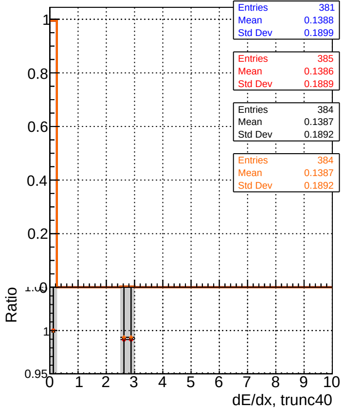
dE/dx estimator 2
