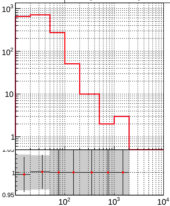
RecoAssoc2GenPVM
