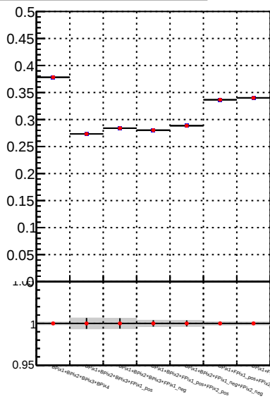
Fake rate vs. DQM TT mkFit-DQM_pless_orig DQM TT mkFit-DQM_pless_mod
