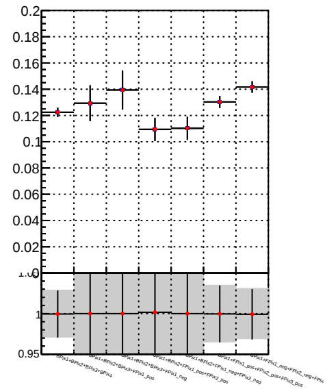
Fake rate vs. DQM TT mkFit-DQM_pless_orig DQM TT mkFit-DQM_pless_mod
