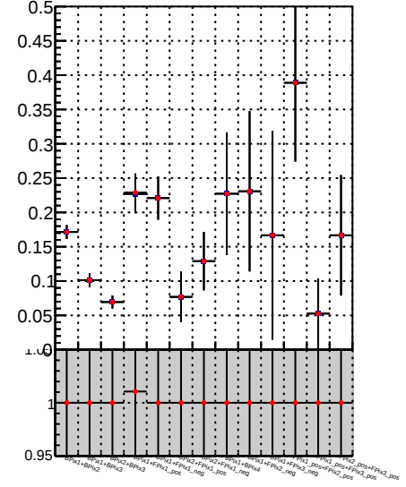
Fake rate vs. — DQM TT mkFit-DQM_pless_orig — DQM TT mkFit-DQM_pless_mod
