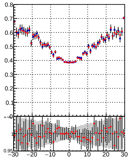
—●— DQM\_TT\_mkFit-DQM\_pless\_orig —●— DQM\_TT\_mkFit-DQM\_pless\_mod
