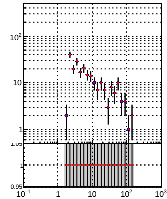
—●— DQM TT mkFit-DQM pless_orig —●— DQM TT mkFit-DQM pless_modi2
