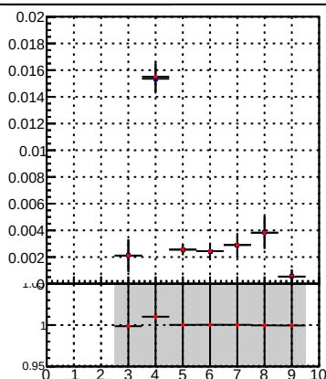
DQM TT mkFit-DQM_pless_orig
