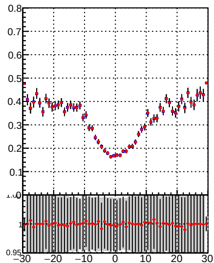
—•— DQM TT mkFit-DQM_pless_orig —•— DQM TT mkFit-DQM_pless_modi
