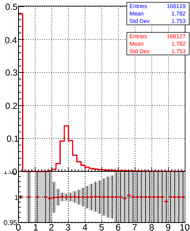
dE/dx estimator 2
