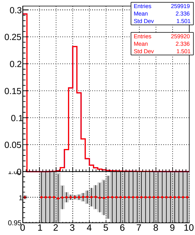
dE/dx estimator 1
