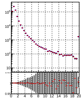
Legend: DQM TT mkFit-DQM_pless_orig DQM TT mkFit-DQM_pless_modi
