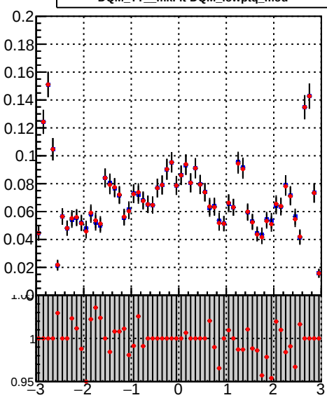
DQM\_TT\_mkFit-DQM\_lowptq\_orig DQM\_TT\_mkFit-DQM\_lowptq\_mod
