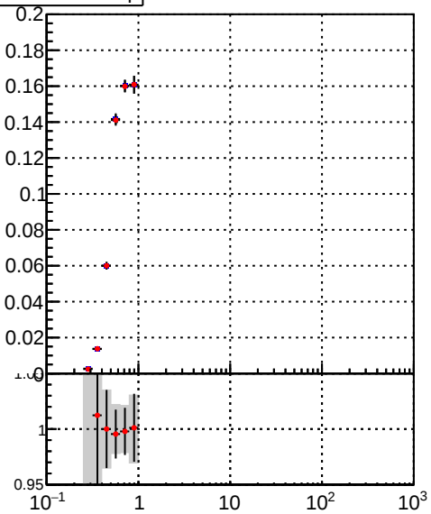
DQM\_TT\_mkFit-DQM\_lowptq\_orig DQM\_TT\_mkFit-DQM\_lowptq\_mod
