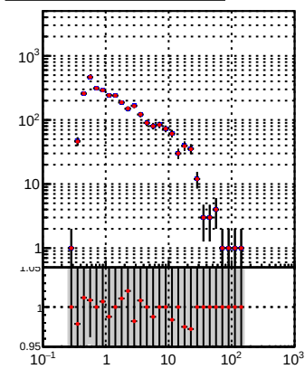
—•— DQM TT mkFit-DQM_lowptq_orig —•— DQM TT mkFit-DQM_lowptq_mod
