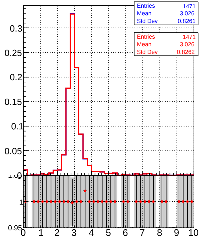
dE/dx estimator 2
