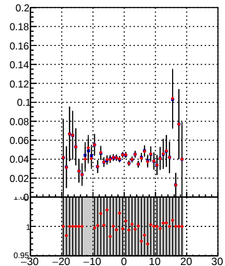
—•— DQM TT mkFit-DQM_lowptq_orig —•— DQM TT mkFit-DQM_lowptq_modi3
