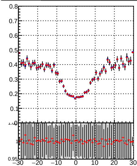
—●— DQM\_TT\_mkFit-DQM\_lowptq\_orig —●— DQM\_TT\_mkFit-DQM\_lowptq\_modi3
