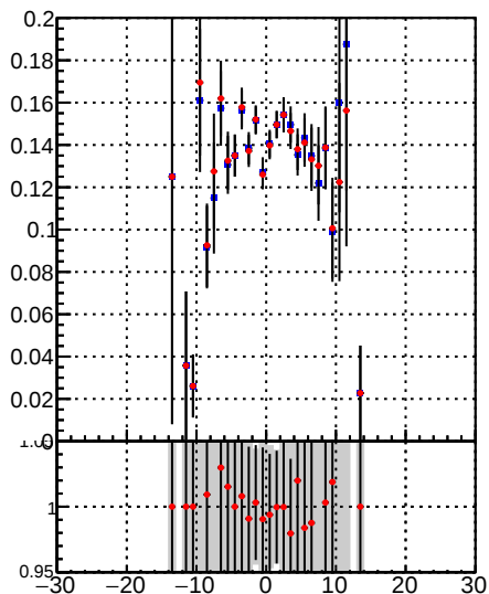
—•— DQM TT mkFit-DQM_lowptq_orig —•— DQM TT mkFit-DQM_lowptq_mod3
