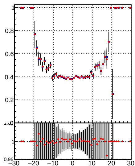
—•— DQM TT mkFit-DQM_lowptq_orig —•— DQM TT mkFit-DQM_lowptq_modi3
