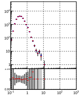
DQM TT mkFit-DQM_lowptq_orig DQM TT mkFit-DQM_lowptq_modi3
