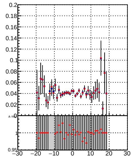
—•— DQM TT mkFit-DQM_lowptq_orig —•— DQM TT mkFit-DQM_lowptq_mod12
