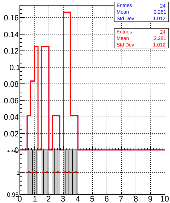
dE/dx estimator 1
