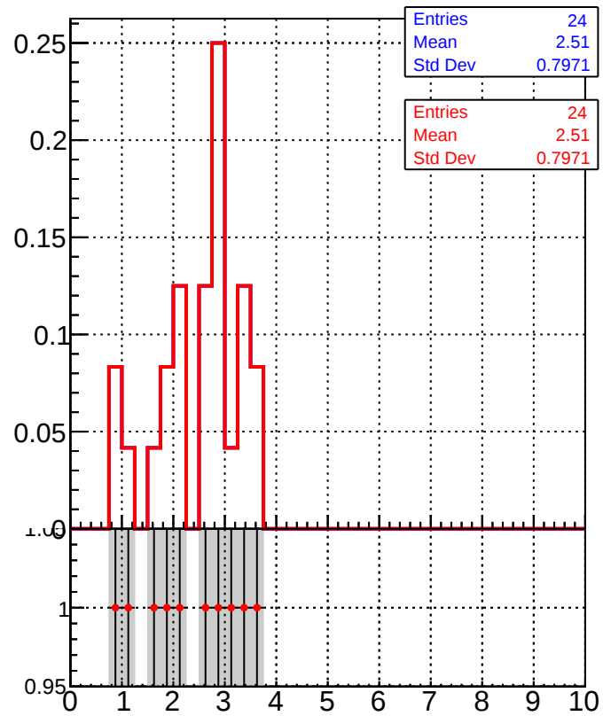
dE/dx estimator 2
