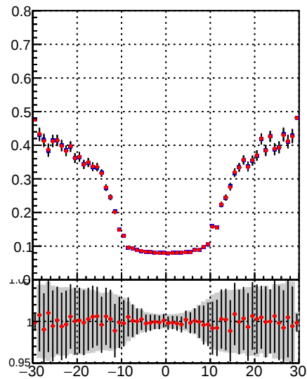
—●— DQM\_TT\_mkFit-DQM\_lowptq\_orig —●— DQM\_TT\_mkFit-DQM\_lowptq\_modi2
