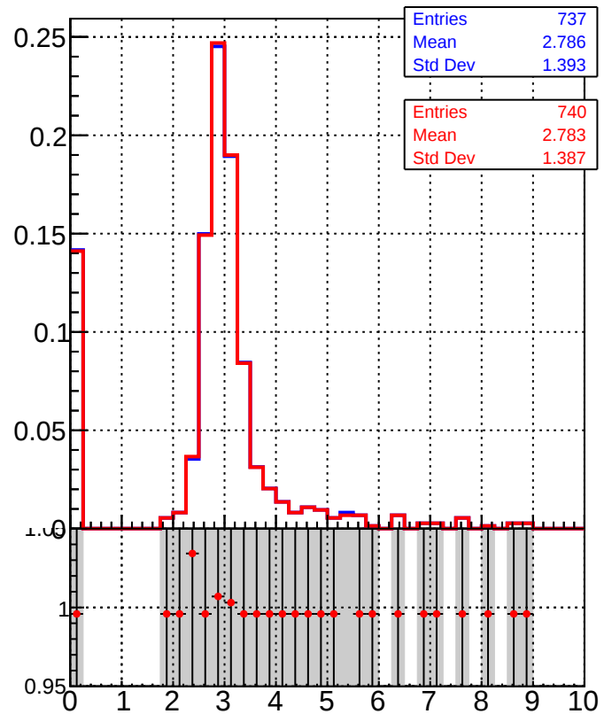
dE/dx estimator 2
