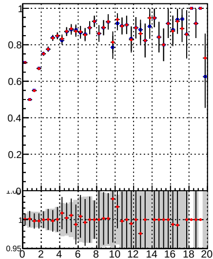
Fake rate vs. \chi^2 DQM TT mkFit-DQM_lowptq_orig \chi^2 DQM TT mkFit-DQM_lowptq_modI2
