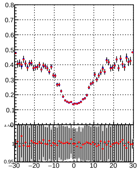
—●— DQM TT mkFit-DQM_lowptq_orig —●— DQM TT mkFit-DQM_lowptq_mod12
