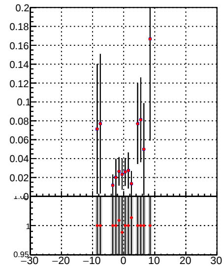
—•— DQM TT mkFit-DQM_lowptq_orig —•— DQM TT mkFit-DQM_lowptq_modi2
