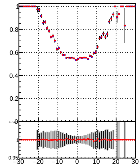
—•— DQM TT mkFit-DQM_lowptq_orig —•— DQM TT mkFit-DQM_lowptq_mod2
