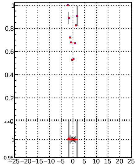
—•— DQM TT mkFit-DQM_lowptq_orig —•— DQM TT mkFit-DQM_lowptq_mod2
