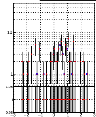
N of reco track vs \eta pT eta —•— DQM TT mkFit-DQM_lowptq_orig —•— DQM TT mkFit-DQM_lowptq_modi2
