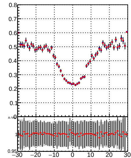
—•— DQM\_TT\_mkFit-DQM\_lowptq\_orig —•— DQM\_TT\_mkFit-DQM\_lowptq\_modI2
