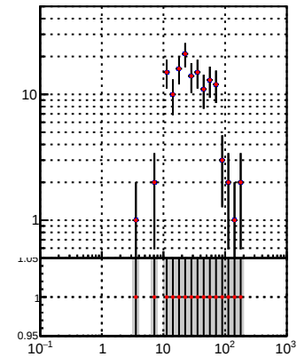
—•— DQM TT mkFit-DQM_lowptq_orig —•— DQM TT mkFit-DQM_lowptq_modi
