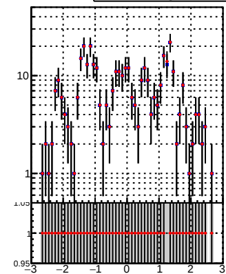
—•— DQM TT mkFit-DQM_lowptq_orig —•— DQM TT mkFit-DQM_lowptq_modi
