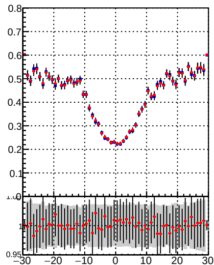
—●— DQM TT mkFit-DQM_init_orig —●— DQM TT mkFit-DQM_init_mod
