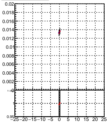
■ DQM_TT_mkFit-DQM_init_orig ■ DQM_TT_mkFit-DQM_init_mod
