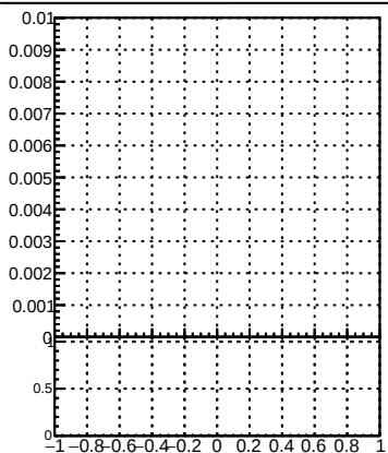
DQM_TT_mkFit-DQM_init_mod
