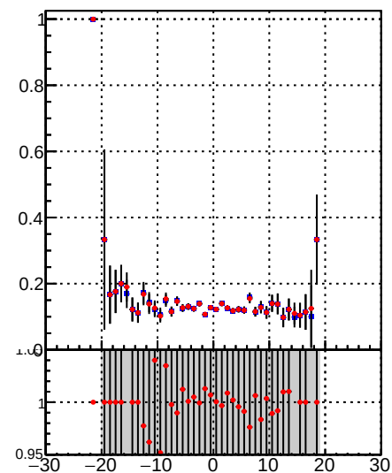
Fake rate vs d —•— DQM TT mkFit-DQM_init_orig —•— DQM TT mkFit-DQM_init_mod
