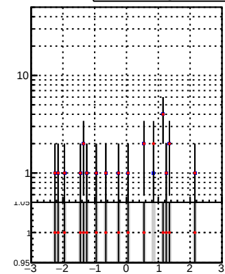
N of reco track vs \eta pT eta —•— DQM_TT_mkFit-DQM_init_orig —•— DQM_TT_mkFit-DQM_init_mod
